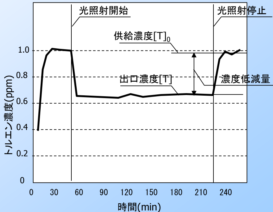
試験結果例
