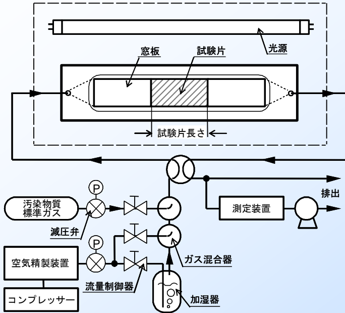
試験装置
