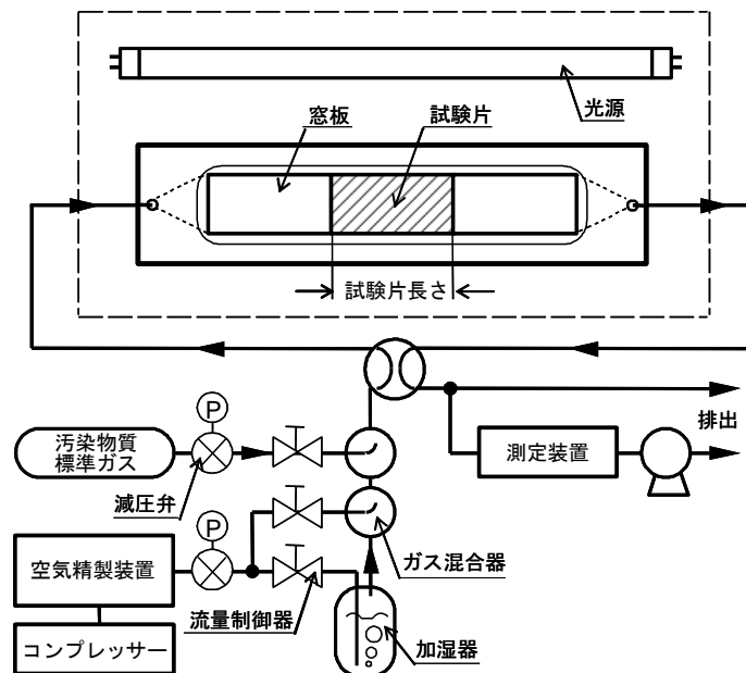
図1 JIS R1701 シリーズ試験装置図
