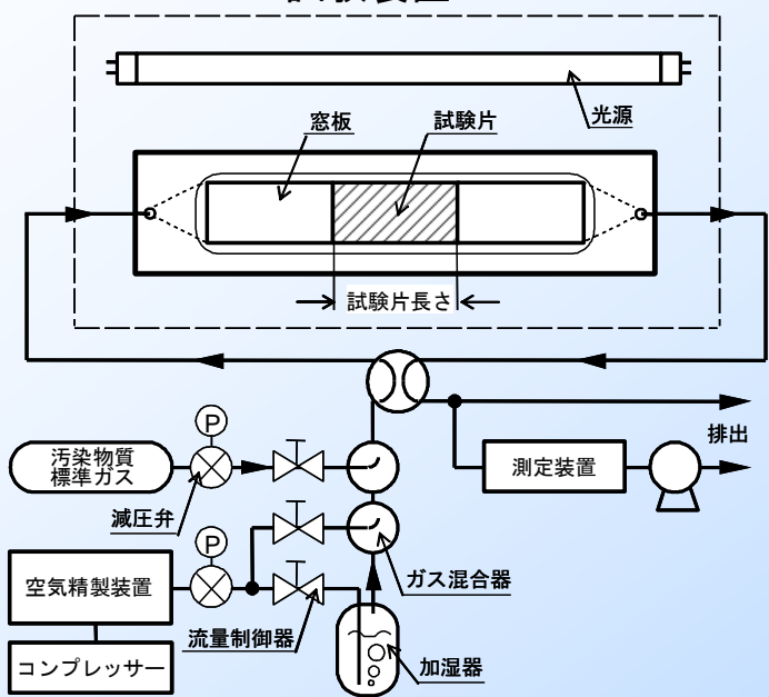
試験装置
