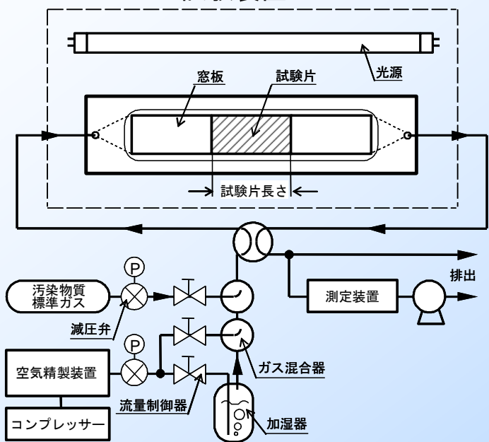
試験装置
